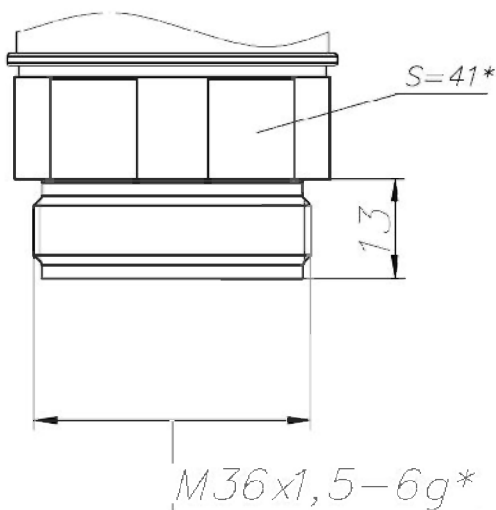
Рисунок Г.3 — Габаритные размеры штуцера преобразователей с кодом присоединительной части А
