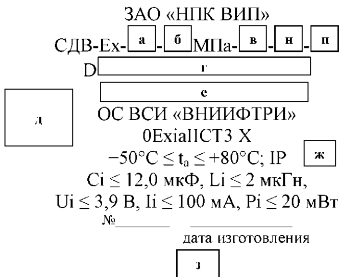
Рисунок Б.11 — Маркировка на корпусе преобразователей СДВ-Ех с маркировкой взрывозащиты «0ExiaIICT5 X»
